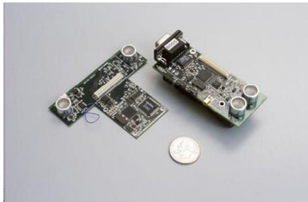
微型控制器 Cricket
